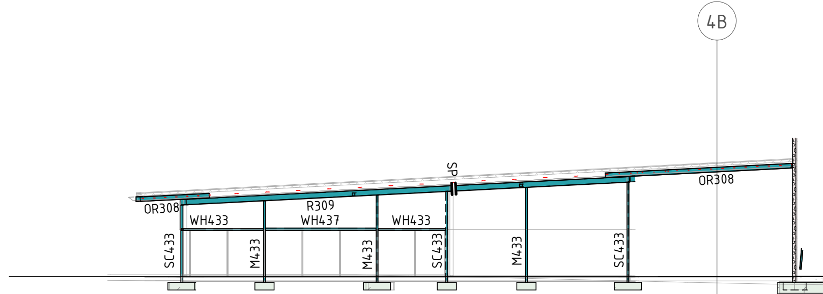
SECTION B3 SCALE 1 : 200
